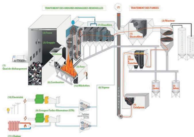
Schéma du process simplifié d'une ligne d'incinération
